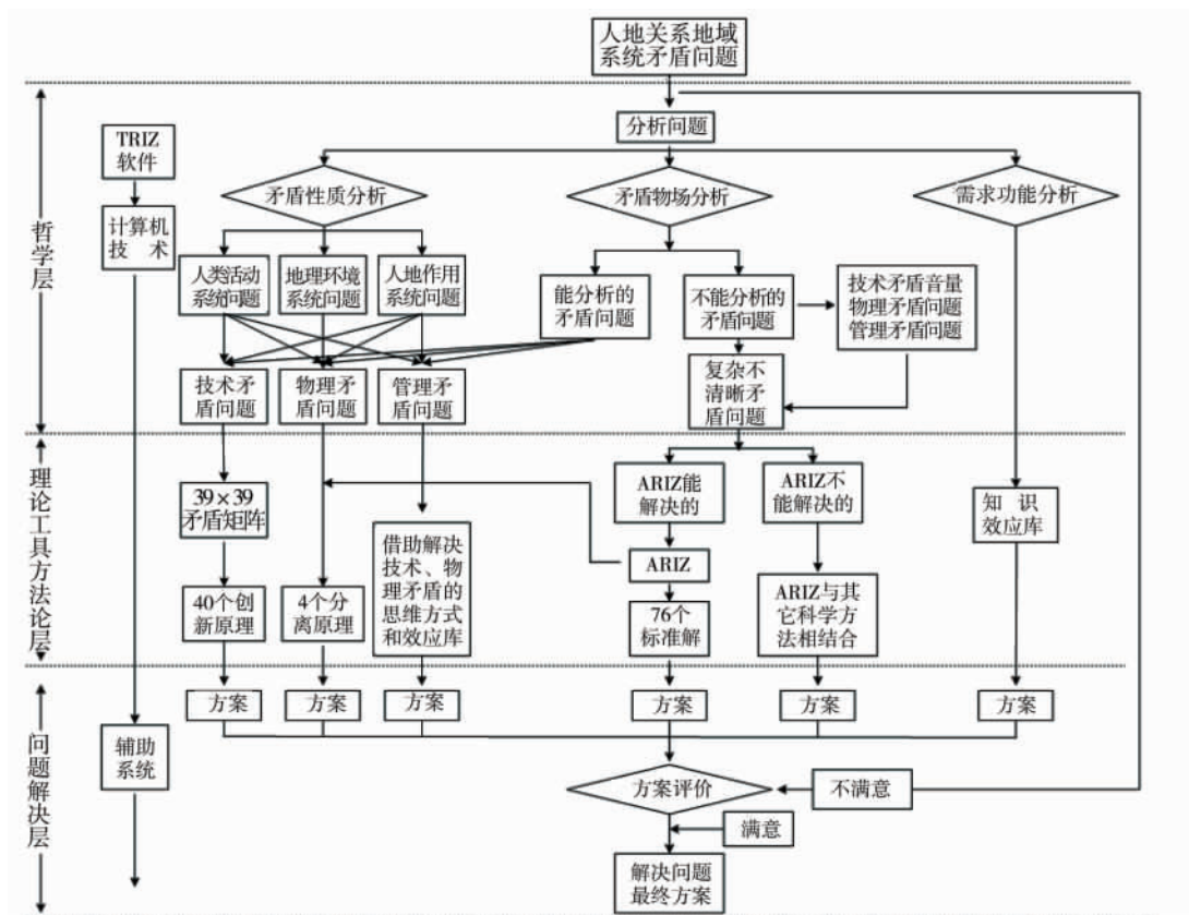
图3 TRIZ 解决人地关系问题的逻辑范式
