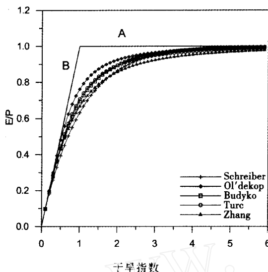
图 1 不同蒸发率函数比较
