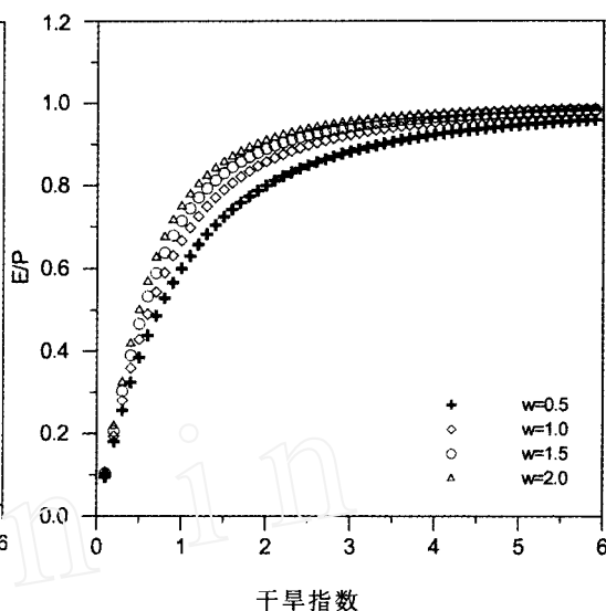
图 2 不同植被有效水系数的蒸发率函数曲线
