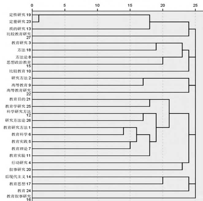
图3 聚类分析树状图
