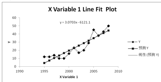
图 2 一元线性回归分析图
